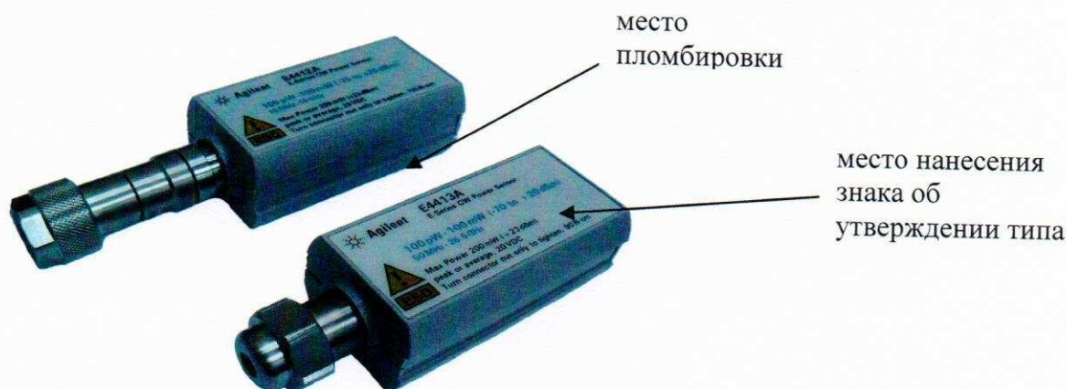
Рисунок 1 – Внешний вид преобразователей измерительных E4412A, E4413A
